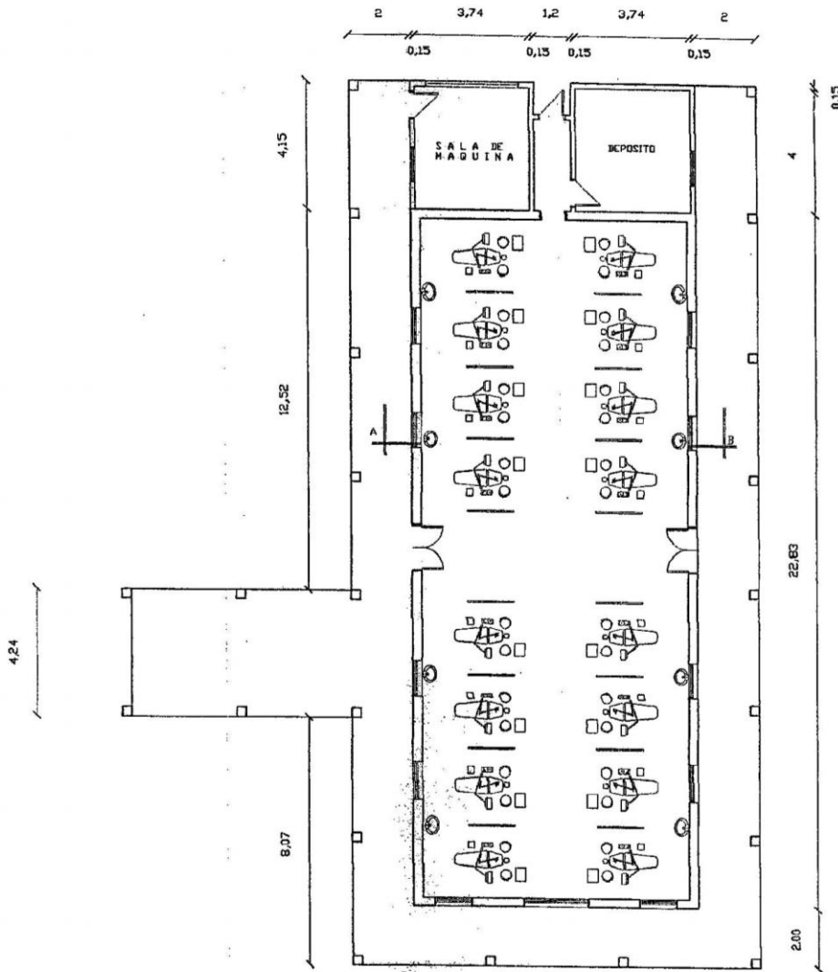
PLANTA ARQUITECTONICA
