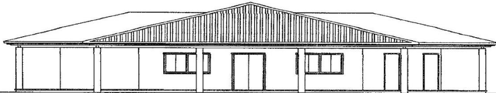
FACHADA PRINCIPAL Esc. 1/75
